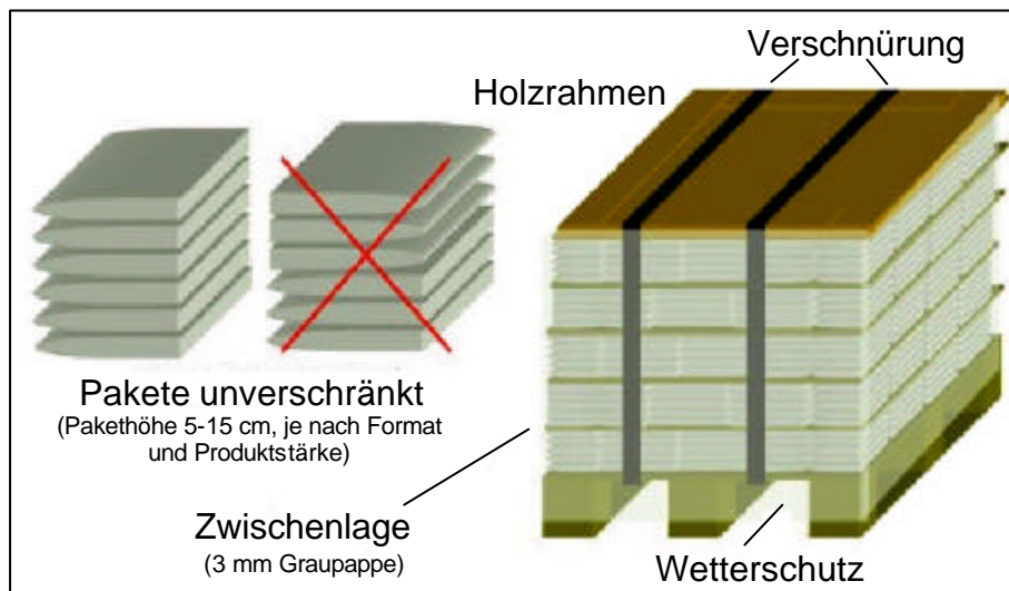
Abb.: Palettenverpackung
